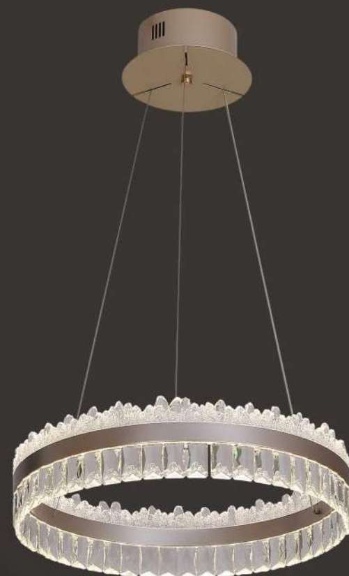
型号: 69631-500/600 材质: 优质铝材+国产一级水晶+亚克力 规格: \Phi 500mm LED*48 双色 规格: \Phi 600mm LED*63 双色
