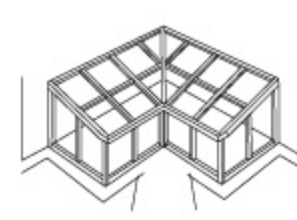
位于房屋内角的阳光房 Sunroom attached inside angle of the house
