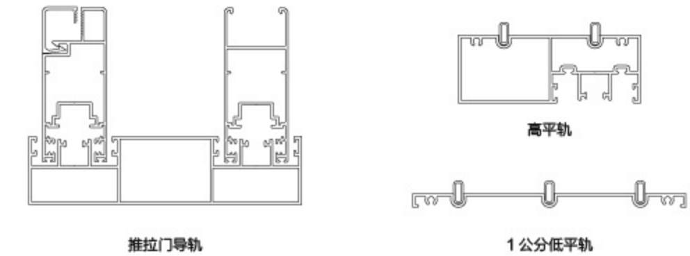
导轨示意图 Track schematic diagram
