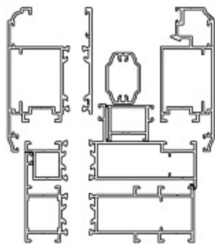
产品结构图 Product Structure Diagram
