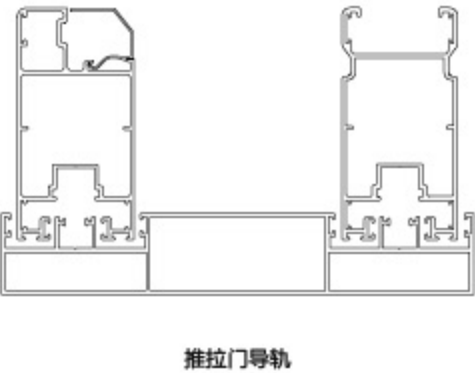
导轨示意图 Track schematic diagram
