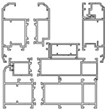
产品结构图 Product Structure Diagram
