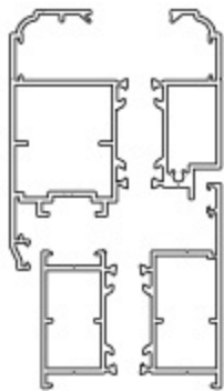
产品结构图 Product Structure Diagram
