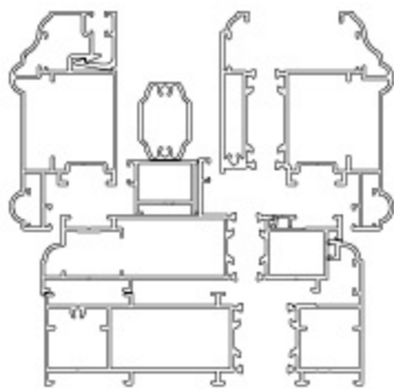
产品结构图 Product Structure Diagram
