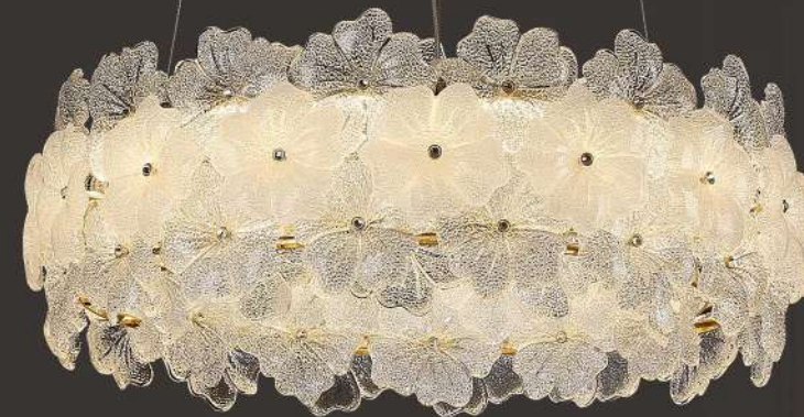
型号: 69689-500/600 材质: 优质五金+国产一级玻璃 规格: \Phi 500*H260\text{mm} LED*63W双色 规格: \Phi 600*H260\text{mm} LED*72W双色
