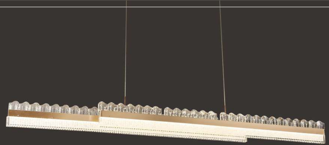
型号：69578-直条 材质：优质铝材+国产一级水晶+亚克力 规格：1200*H100mm 光源：LED*30W 双色
