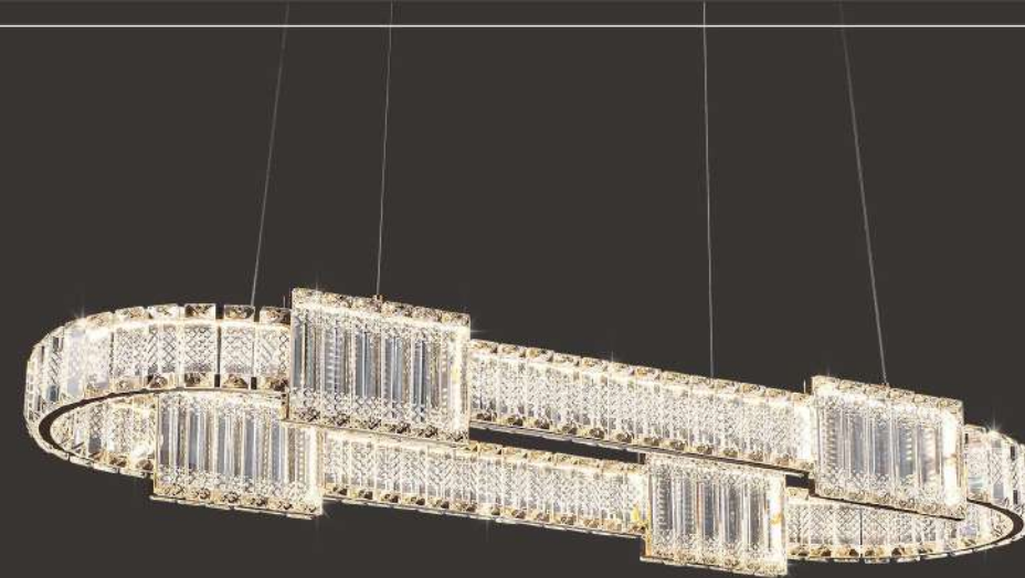
型号: 69350-900 椭圆 材质: 优质五金+国产一级水晶 规格: 900*H300\text{mm} 光源: LED*70W 双色
