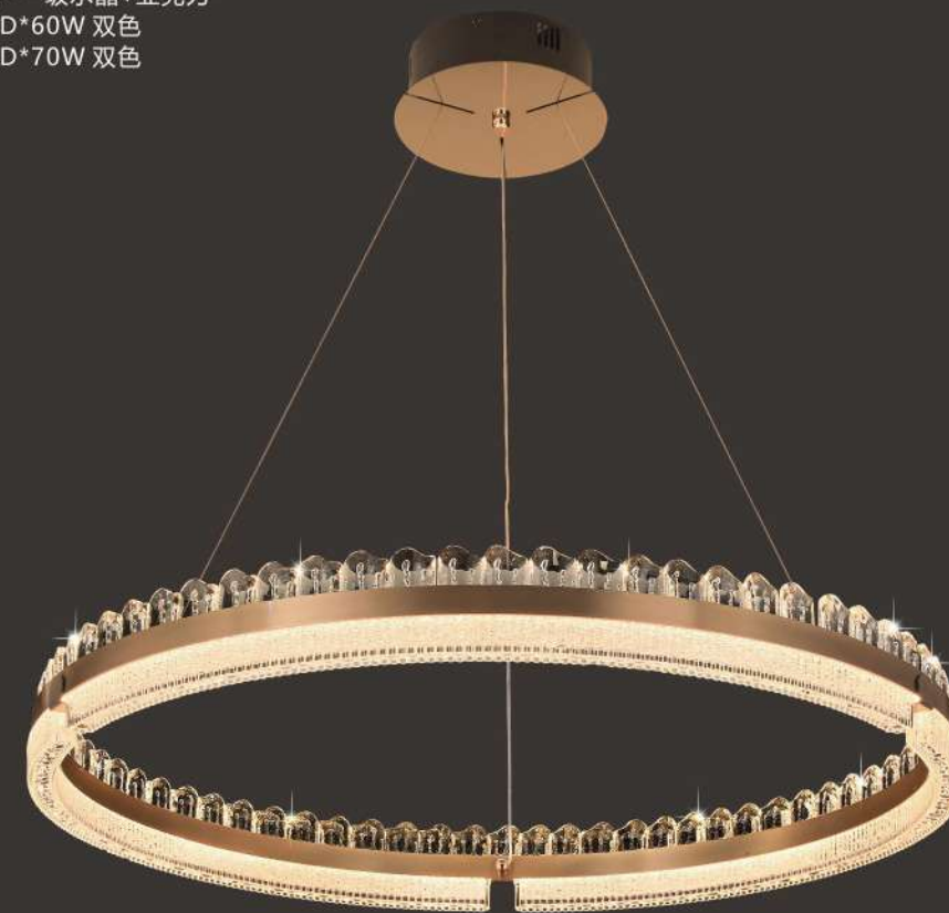
型号: 69578-800 材质: 优质铝材+国产一级水晶+亚克力 规格: \Phi 800\text{mm} 光源: LED*108W 双色
