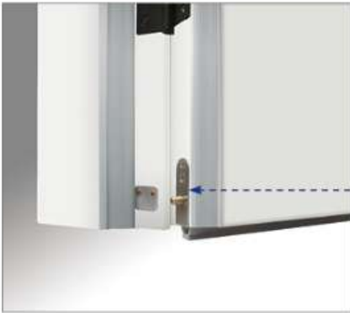
升降静音密封条 门扇底部使用升降静音密封条，关闭木门时密封条会下降，具有隔音、防尘、防虫功能。
