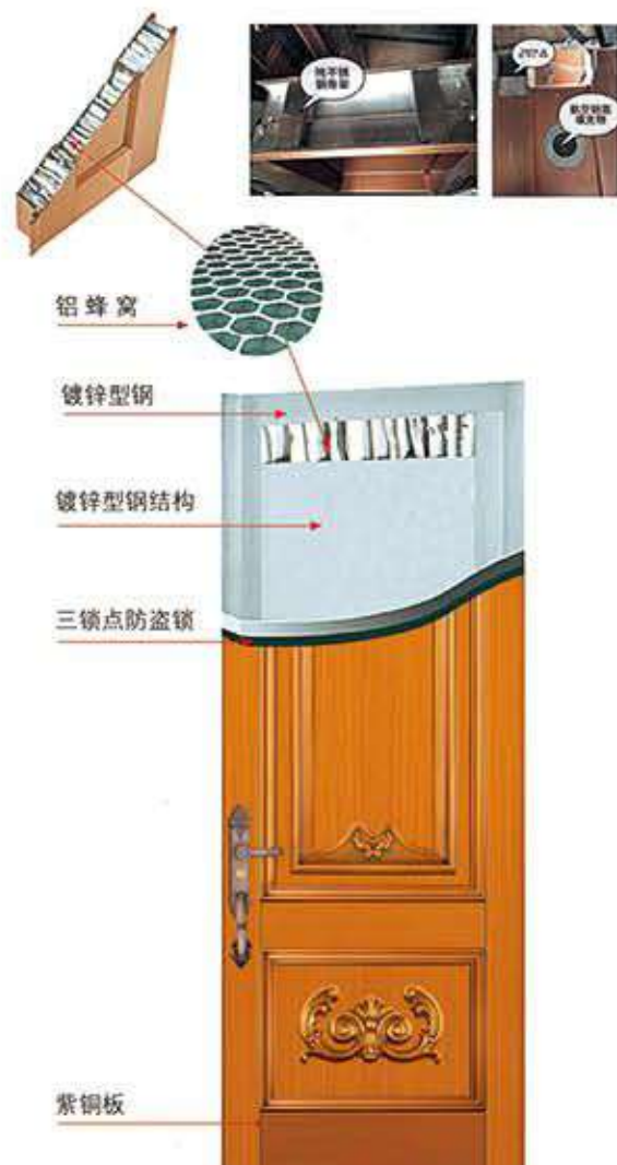
铜门内结构示意图
